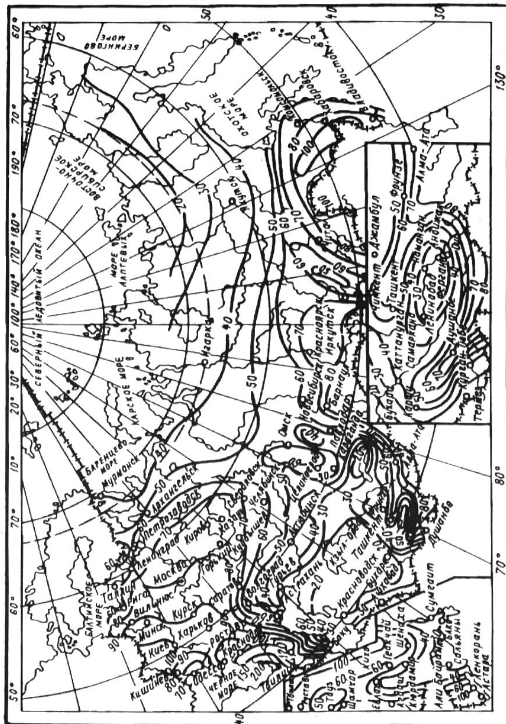
Чертеж 1. Значения величин интенсивности дождя q_{20}
