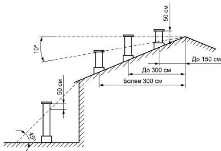
Рисунок Г.1 - Схема вывода дымовых каналов на крышу здания
